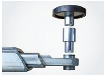
Hohe Flexibilität und Sicherheit durch Aufnahmeteller-Stecksyst
